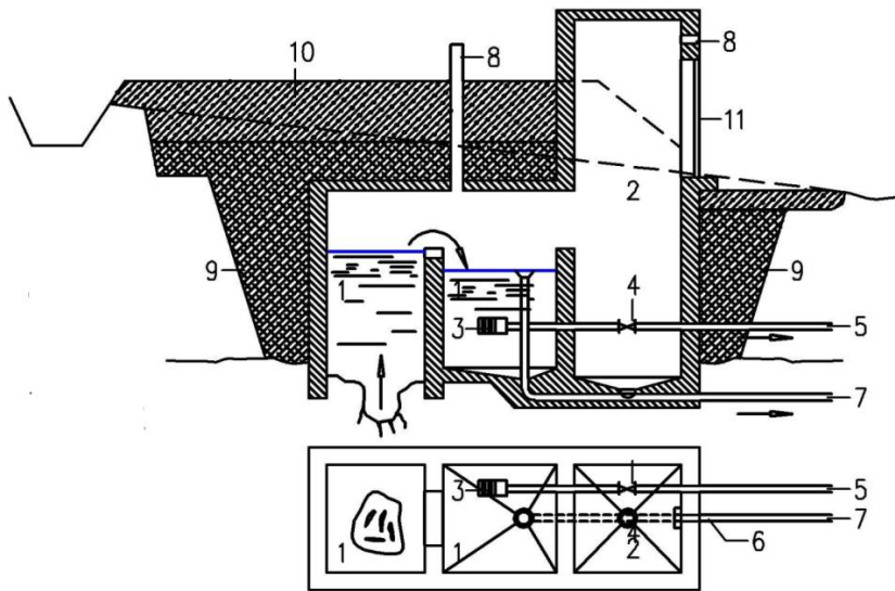
КАПТАЖ НА ВЪЗХОДЯЩ ИЗВОР ( ПЛАН И РАЗРЕЗ )
