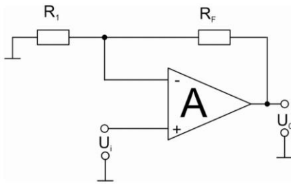
Схема на неинвертиращ усилвател
